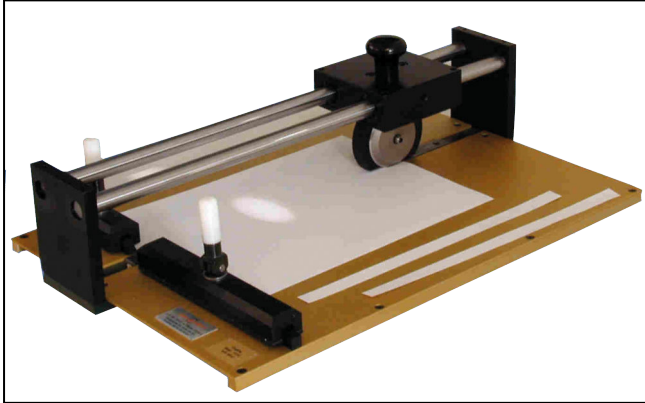
Papierstreifenschneider
